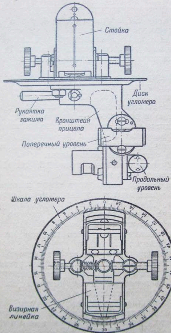
Рис. 13. Прицел (угломер-квадрант)
