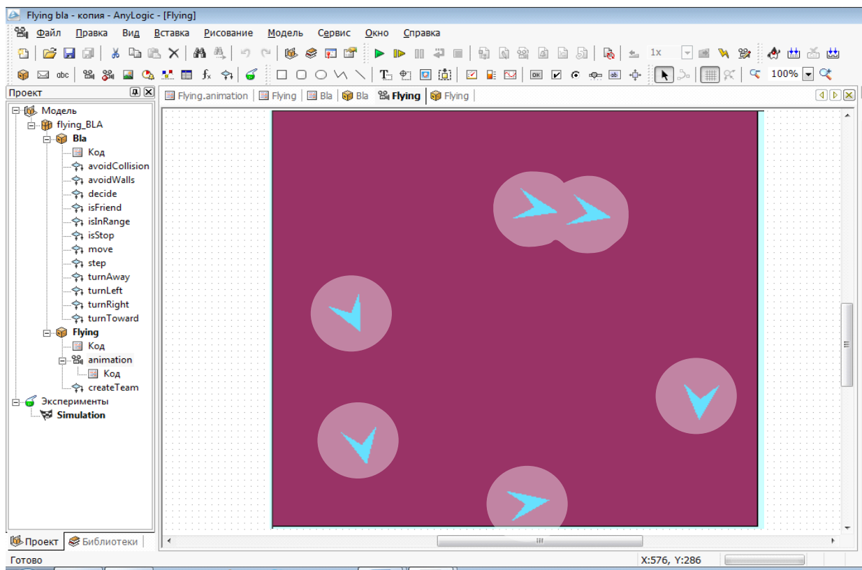
Рис. 2. Имитационная модель
