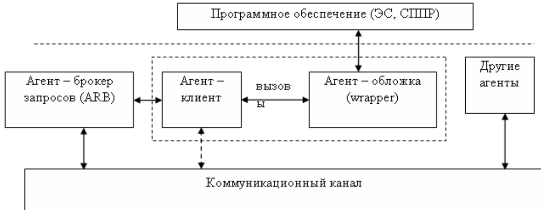
Рис. 3. Схема интеграции агента с существующим программным обеспечением (FIPA '2000)
