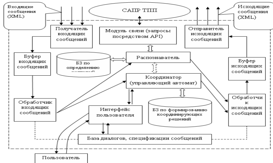
Рис. 4. Функциональная схема автоматной реализации СППР по формированию координирующих решений в сборочном производстве самолетостроительного предприятия
