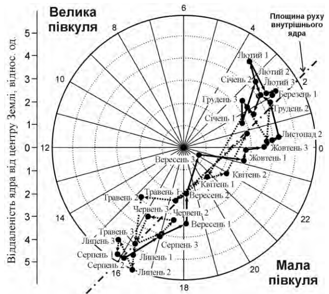
Рис. 2. Траса руху центру внутрішнього ядра усередині Землі протягом року (вид з боку полюсу) [9, 10]
