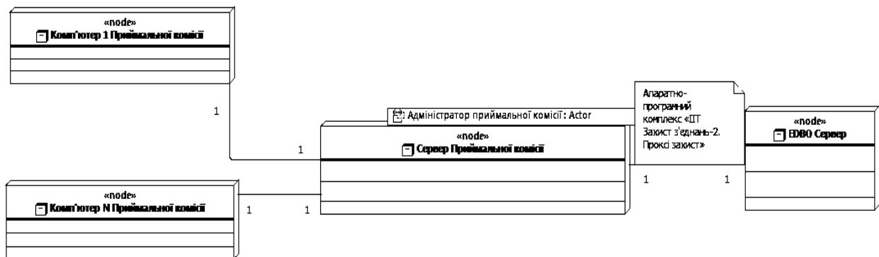
Рис. 1. Фізична діаграма програми
