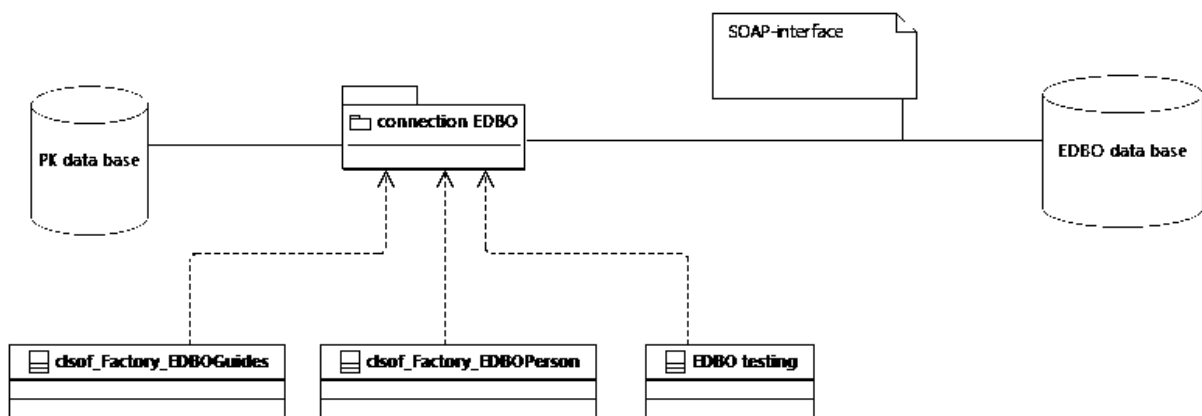
Рис. 2. Функціональна схема програми
