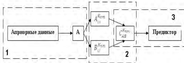
Рис. 2. Загальна схема алгебраїчного підходу к обробці та аналізу даних
