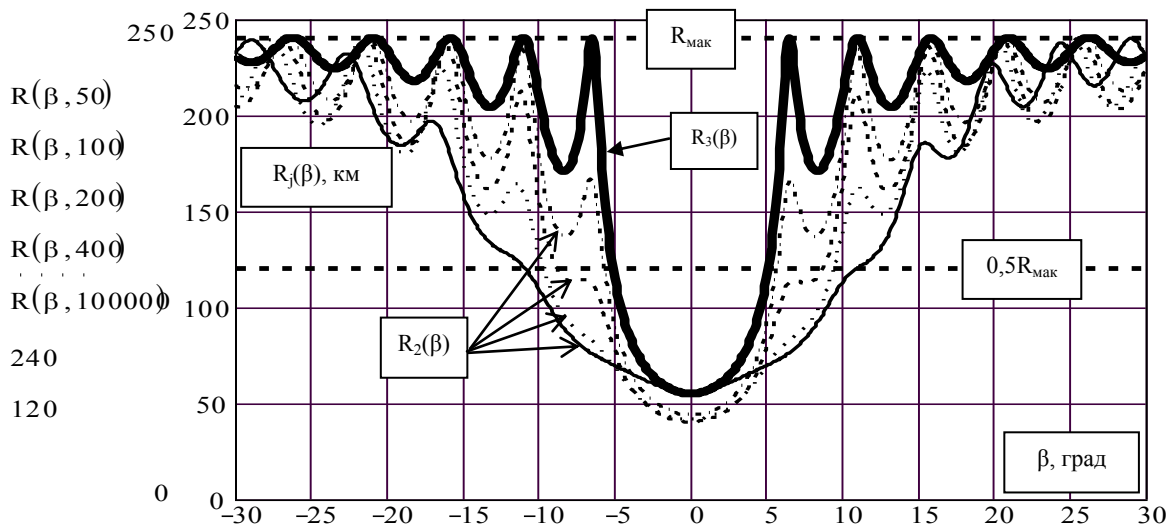
Рис. 3. Фрагмент зоны обнаружения при воздействии на РЛС стандартного ПАП (сплошная толстая кривая) и имитатора помех при его удалении r=50, 100, 200, 400 м (сплошная тонкая, пунктирная, штриховая, штрих-пунктирная кривые соответственно)
