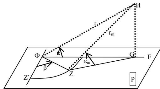
Рис. 2. Взаимное расположение строки с элементами АР (линия \Phi Z ) и имитатора (точка I )
