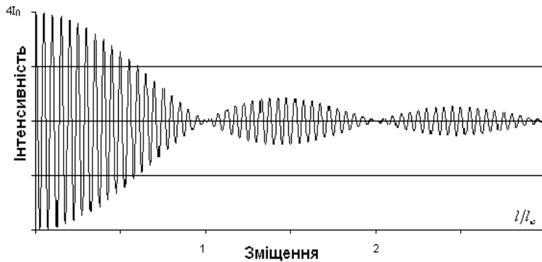
Рис. 2. Залежність інтенсивності інтерференції двох здійснюючих інтерференцій від їхньої різниці ходу l
