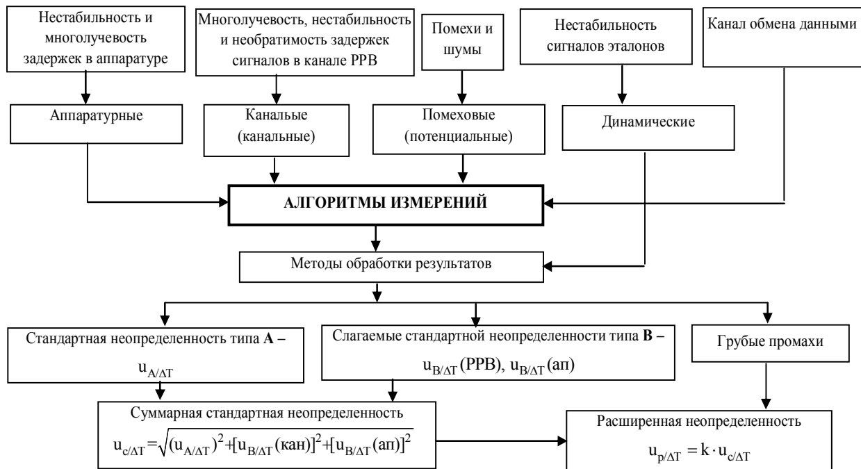
Рис. 2. Структура погрешностей и неопределенности сличения с использованием сигналов ГС
