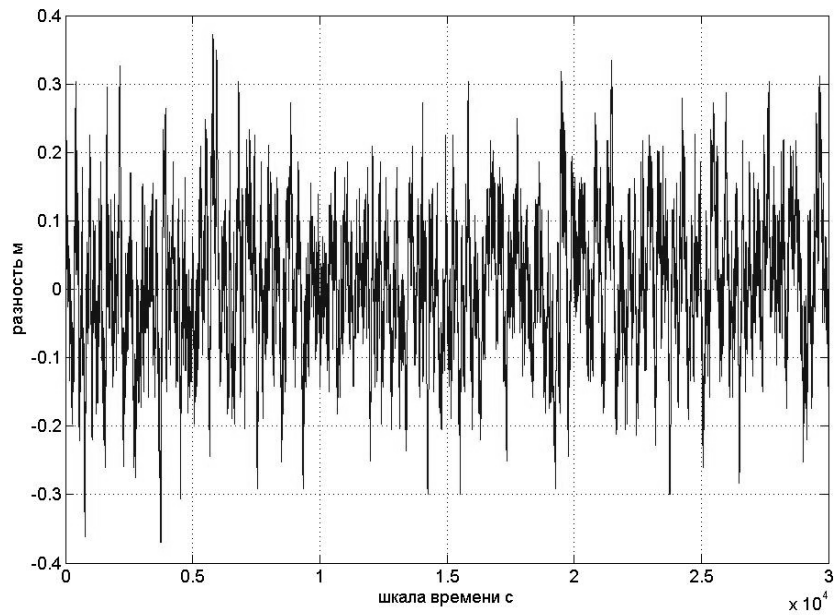
Рис. 6. Разность псевдодальностей
