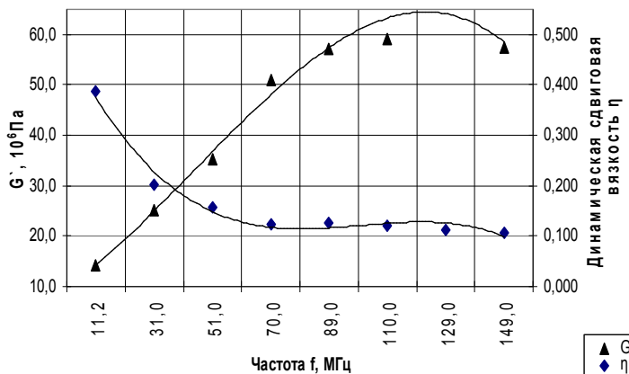
Рис. 3. Частотна залежність динамічних зсувних пружності та в'язкості касторового масла
