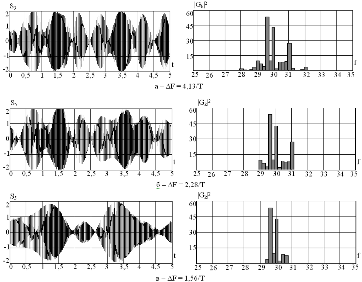
Рис. 2. Вплив обмеження спектра на характеристики послідовності сигналів ансамблю 2f-4φ
