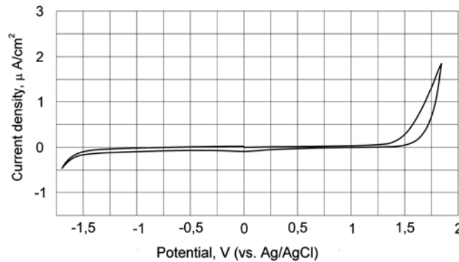
Рис. 4. Циклическая вольтамперограмма 0,1 LiClO 4 в H 2 O на стеклоуглеродной подложке с АПП (установка ELAN-3d при развертке 100 мВ/сек)
