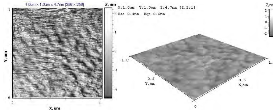
Рис. 3. АСМ изображение поверхности АПП на стеклоуглеродной подложке
