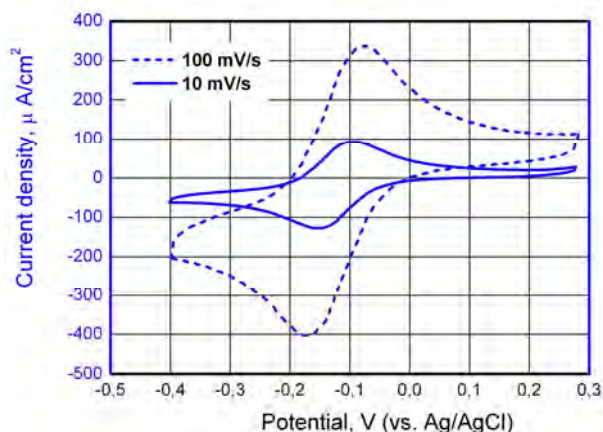
Рис. 7. Циклическая вольтамперограмма редокс-пары 0,94 мМ \{\text{Ru}(\text{NH}_3)_6\}^{+2} / 1,04 мМ \{\text{Ru}(\text{NH}_3)_6\}^{+3} в \text{H}_2\text{O} на фоне 0,1 М \text{NaClO}_4 на электроде из стеклоглуглерода, модифицированном АПП
