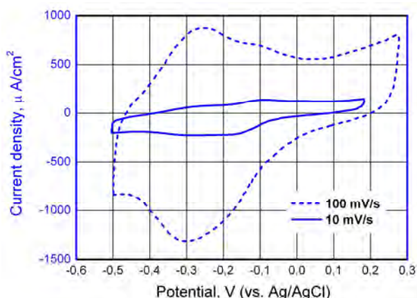
Рис. 6. Циклическая вольтамперограмма редокс-пары 0,94 мМ \{\text{Ru}(\text{NH}_3)_6\}^{+2} / 1,04 мМ \{\text{Ru}(\text{NH}_3)_6\}^{+3} в \text{H}_2\text{O} на фоне 0,1 М \text{NaClO}_4 на электроде из стеклоглуглерода
