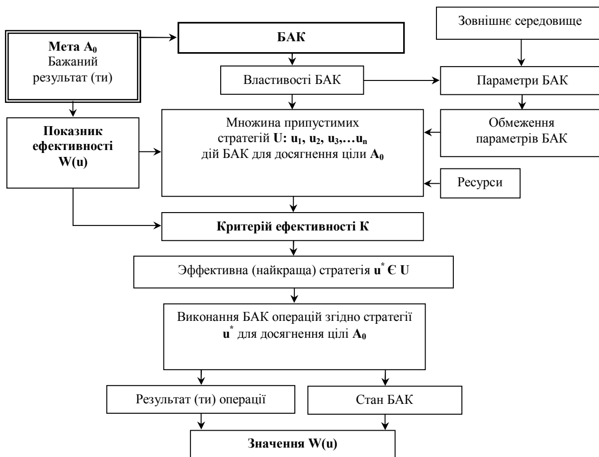
Рис. 4. Загальна структура вибору критеріїв ефективності бойового авіаційного комплексу
