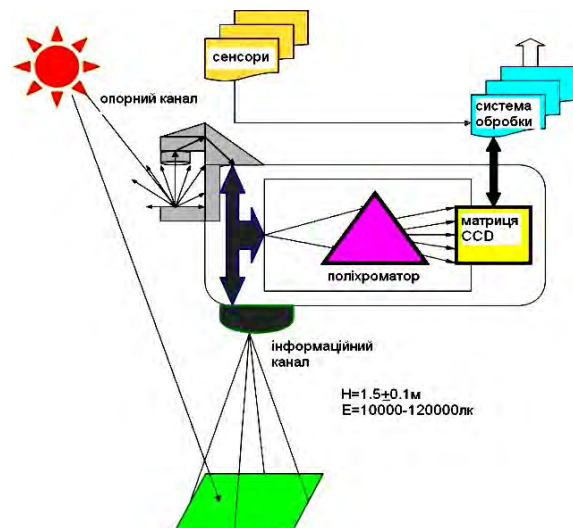
Рис. 1. Блок-схема АПК
