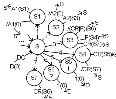
Рис. 5. Граф цикла обмена для команды вида – (A1)(A2)(F)(CR)
