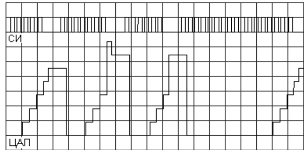
Рис. 8. Диаграмма последовательностей состояний (а) для входной последовательности (б)
