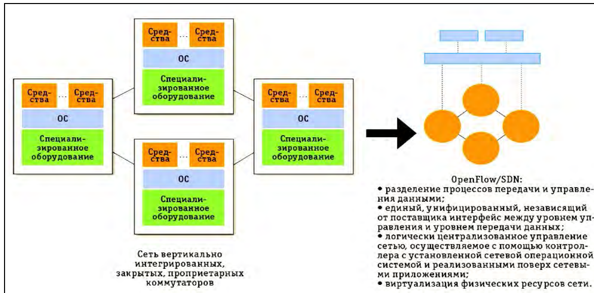
Рис. 3. Задачи OpenFlow
