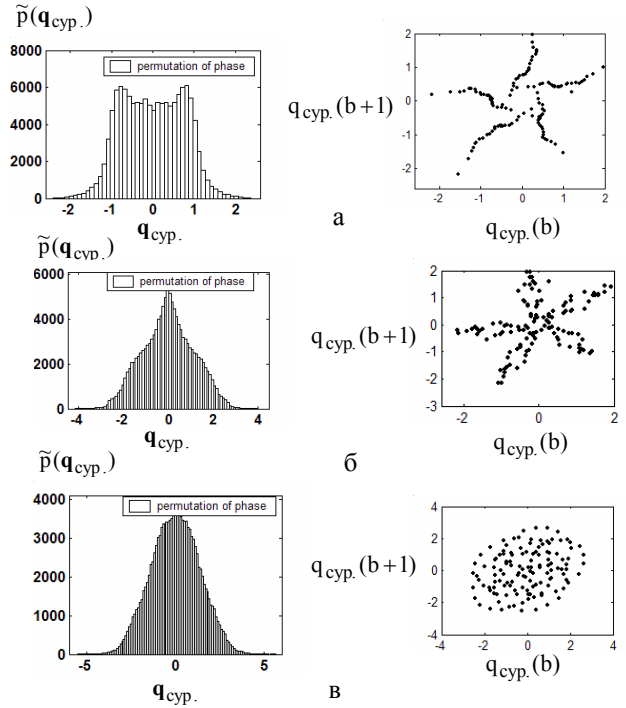
Рис. 3. Гистограммы и фазовые портреты суррогатной помехи при перемешивании фаз Фурье-спектра наблюдений
