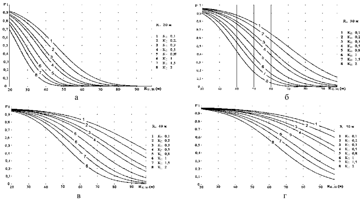
Рис. 4. Вероятности наведения ВТО с ЛГСН на малоразмерную цель в зависимости от расстояния между защищаемым объектом и ложной целью, а также от соотношения интенсивностей сигналов ( K_{п} ) от объекта и от ложной цели для различных значений радиуса поражения R_0
