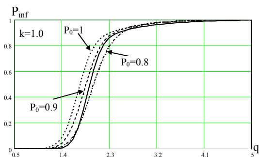
Рис. 3. Залежність P_{inf}=f(k,q,P_0)
