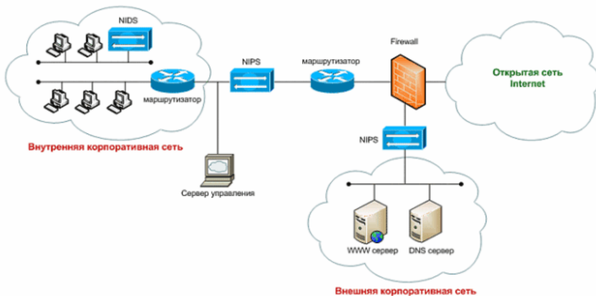
Рис. 1. Типичное размещение сетевых IDS и IPS систем
