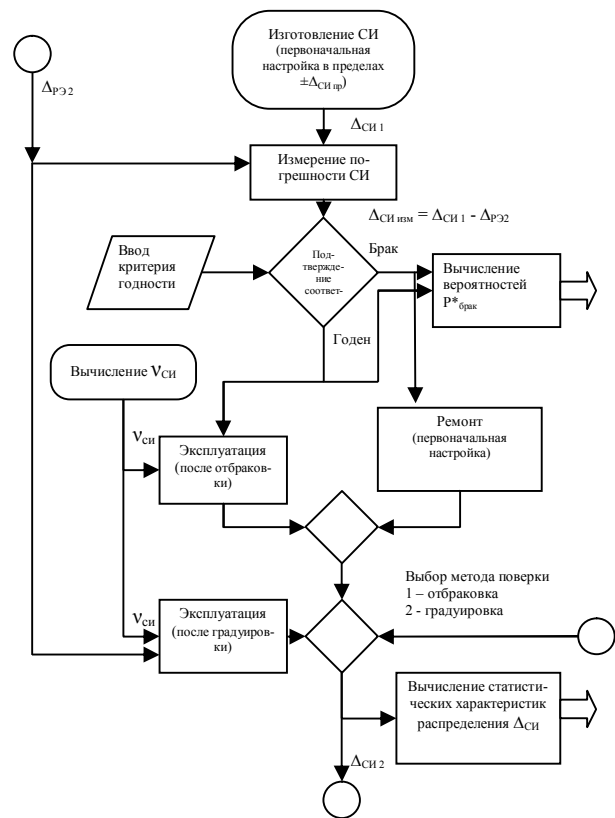
Рис. 2. Блок-схема алгоритма первичной проверки СИ
