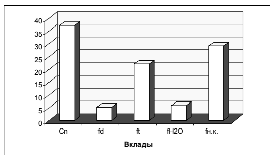
Рис. 2. Доля вклада в суммарную неопределённость измерений массовой концентрации SO 2 в атмосферном воздухе газоанализатором АРМА-370
