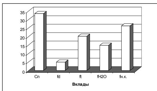
Рис. 1. Доля вклада в неопределённость измерения массовой концентрации CO в атмосферном воздухе газоанализатором АРМА-370
