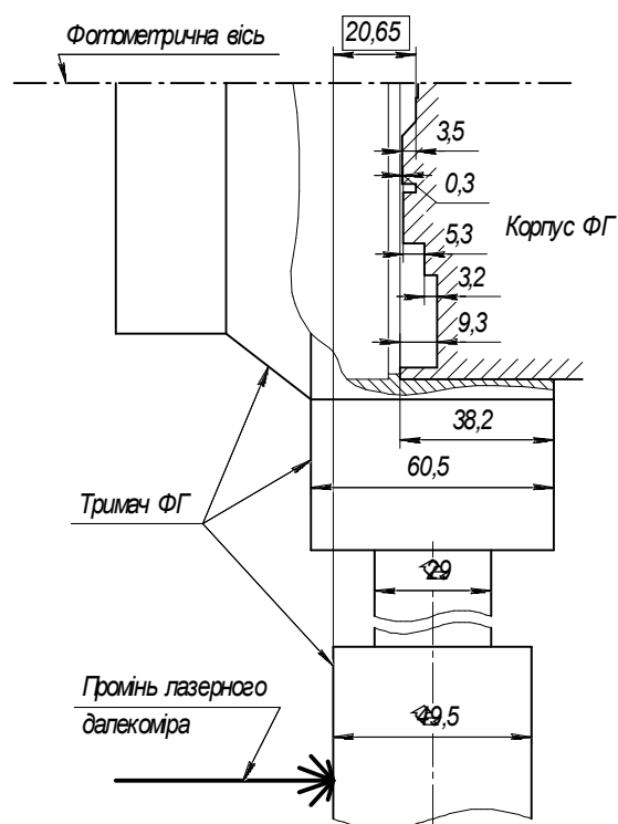
Рис. 2. Перетин фотометричної голівки та тримача
