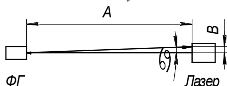
Рис. 3. Положення фотометра (ФГ) та лазера при юстуванні
