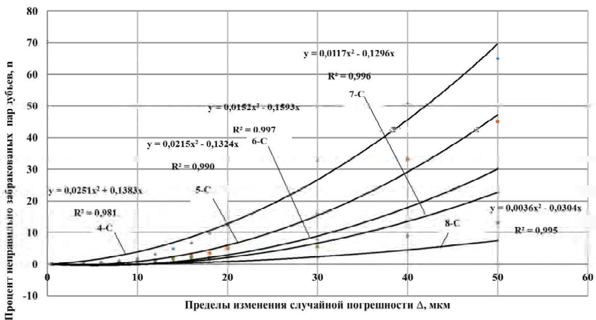
Рис. 3. Зависимости ошибки I рода ( n ) от предельного значения расширенной неопределенности типа А при КТТ = 6
