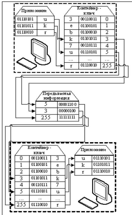
Рис. 1. Схема алгоритма шифрования
