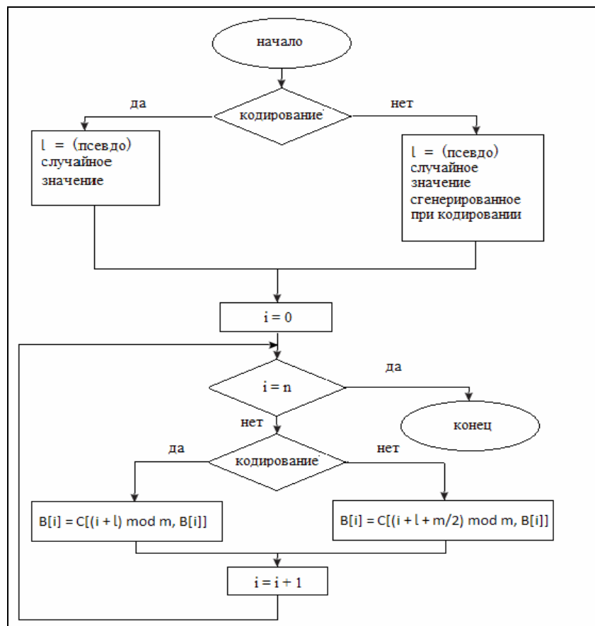
Рис. 2. Блок-схема алгоритма № 1
