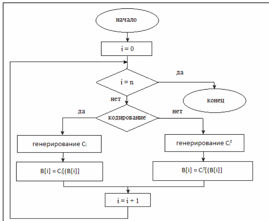
Рис. 3. Блок-схема алгоритма №2
