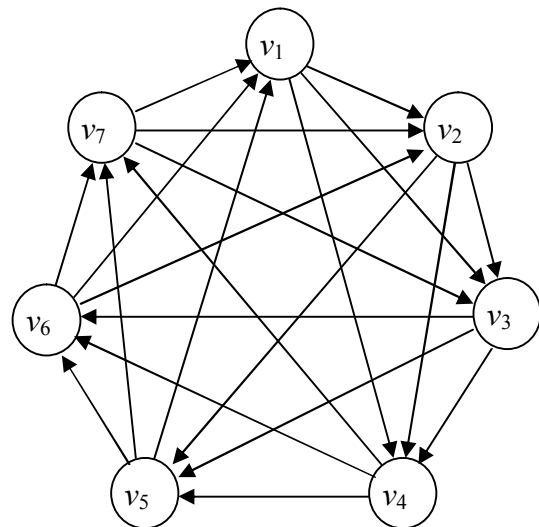
Рис. 3. Розподілене верифікаційне ядро: кожен v_i перевіряє v_{i+1}, v_{i+2}, \dots, v_{i+t} , де t = \lfloor n/2 \rfloor
