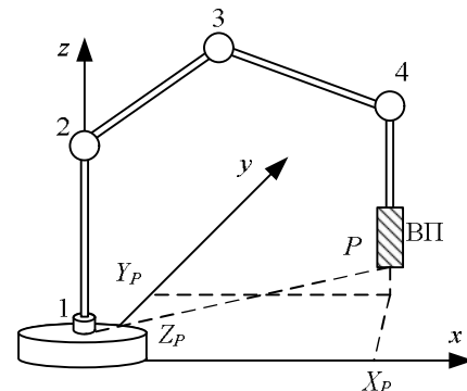
Рис. 2. Механічна система визначення координат із перетворювачами кут повороту – цифровий код
