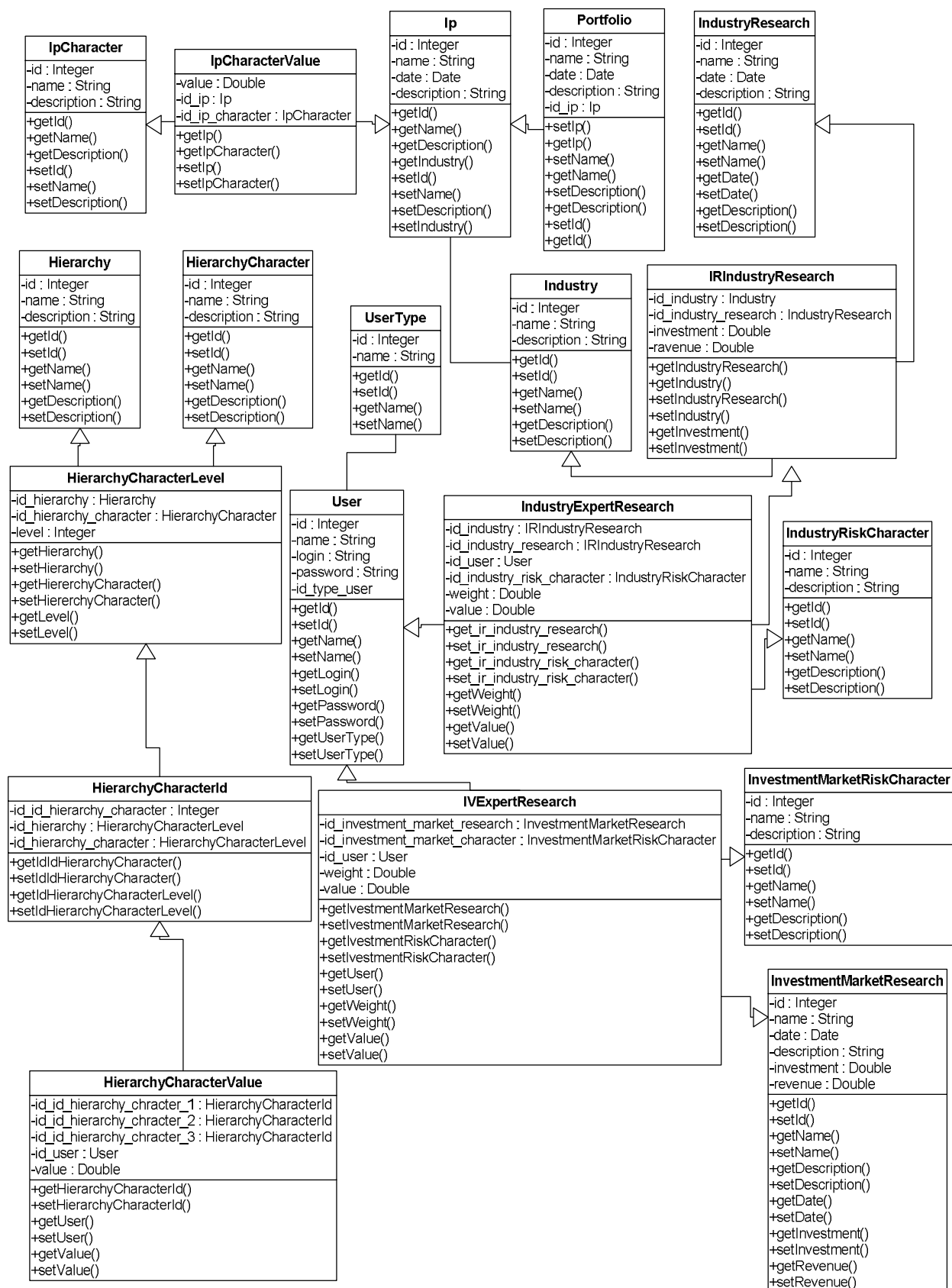
Рис. 4. Діаграма класів програмного комплексу, що реалізує СППР
