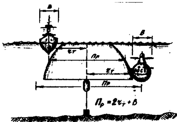
Рис. 2. Зона реагирования неконтактной мины
