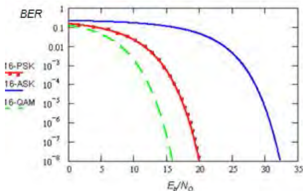
Рис. 2. Энергетическая эффективность модуляций 16-PSK, 16-ASK и 16-QAM
