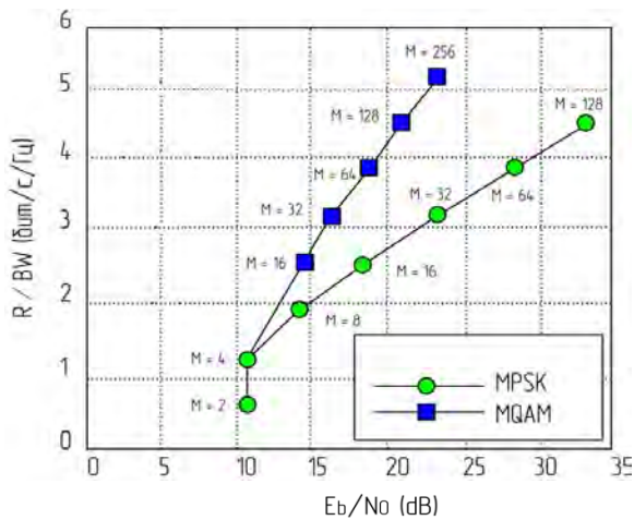
Рис. 5. Спектральна ефективність модуляцій M-QAM і M-PSK
