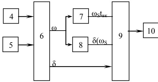
Рис. 2. Схема зонного синхронізатора ( \xi_s = 0 )
