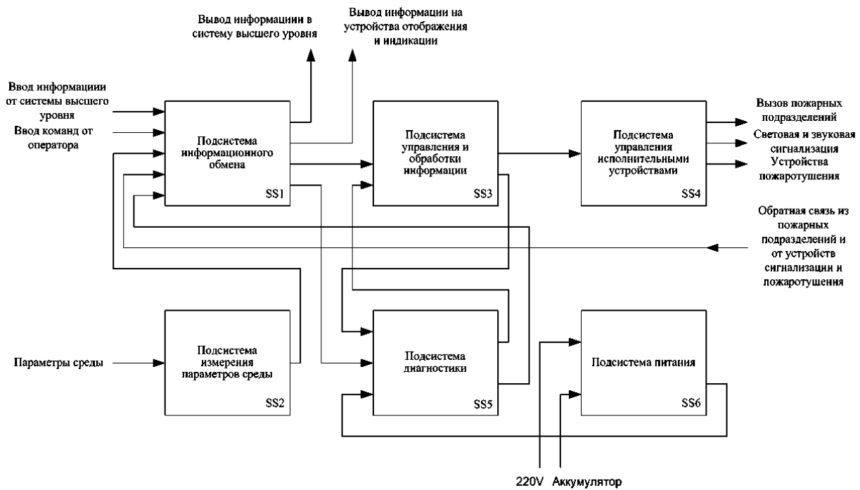
Рис. 1. Структура комп'ютеризованої системи пожежної сигналізації
