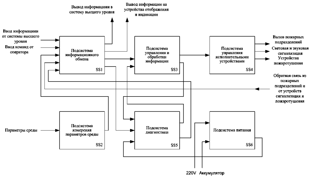
Рис. 1. Структура компьютеризованной системы пожарной сигнализации
