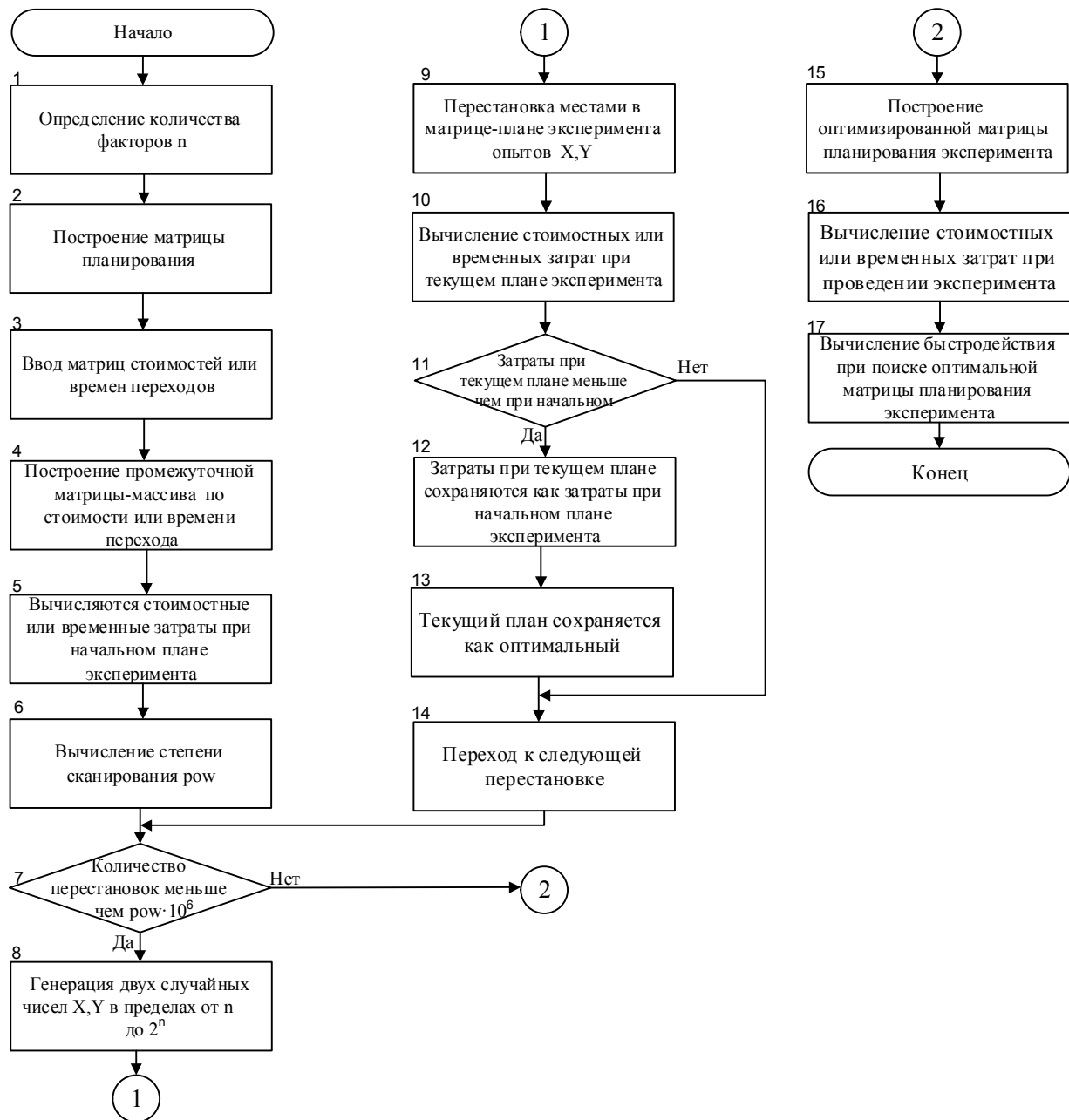
Рис. 1. Схема применения алгоритма имитации отжига для оптимизации многофакторных экспериментов
