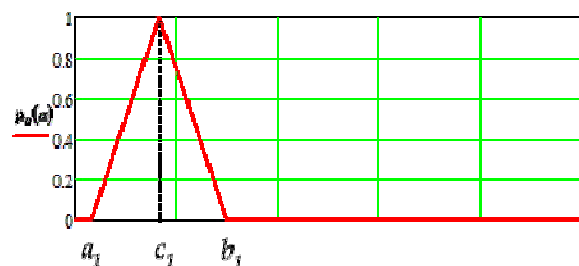
Рис. 1. Функция принадлежности треугольного нечеткого числа a
