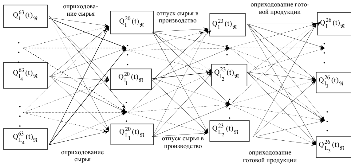
Рис. 1. Граф последовательности отображения подмножеств анализа при проверке предпосылки «полнота»
