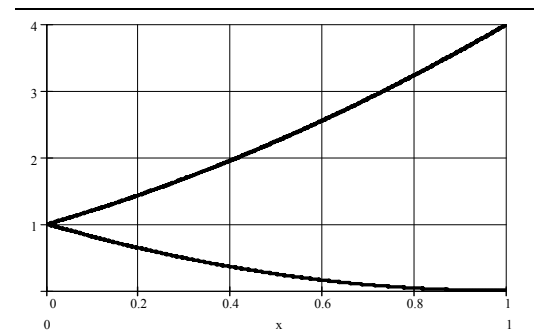
Рис. 3. Графіки функцій f_3 та f_4 при 0 < A_{v_B} < 1
