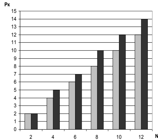
Рис. 3. Збільшення кількості ракетних каналів ЗРК при використанні методу розподілу енергетичного ресурсу БФ РЛС в режимі наведення ЗРК
