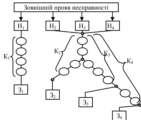
Рис. 1. Структурна схема усунення несправностей: Н – несправність; Р – апіорна ймовірність появу несправності; ПРО – елементарна операція; ДО – комплекс розбірно-складальних елементарних операцій; З – необхідна запасна частина для заміни несправної деталі (вузла) на справну
