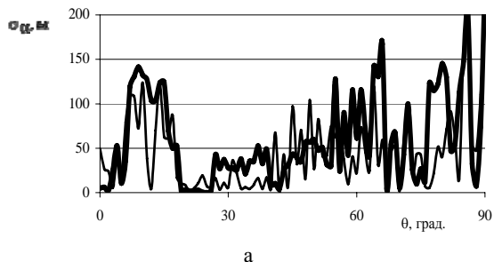
Рис. 5. Розподіл величини \sigma_{II} для моделі АС з обтічником ЗКР III, узгодженим на нормальне падіння
