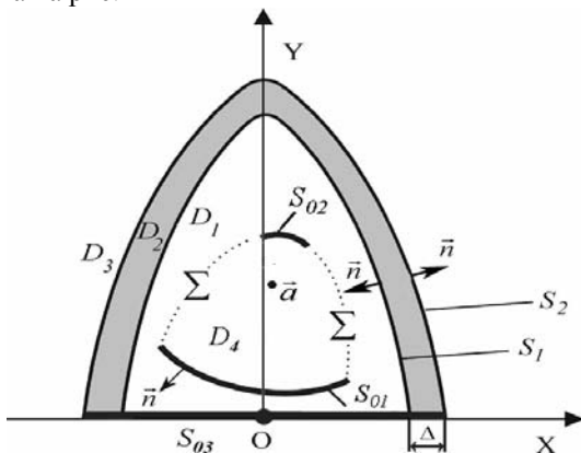
Рис. 2. Двомірна модель дводзеркальної АС, яка вкрита діелектричним обтічником
