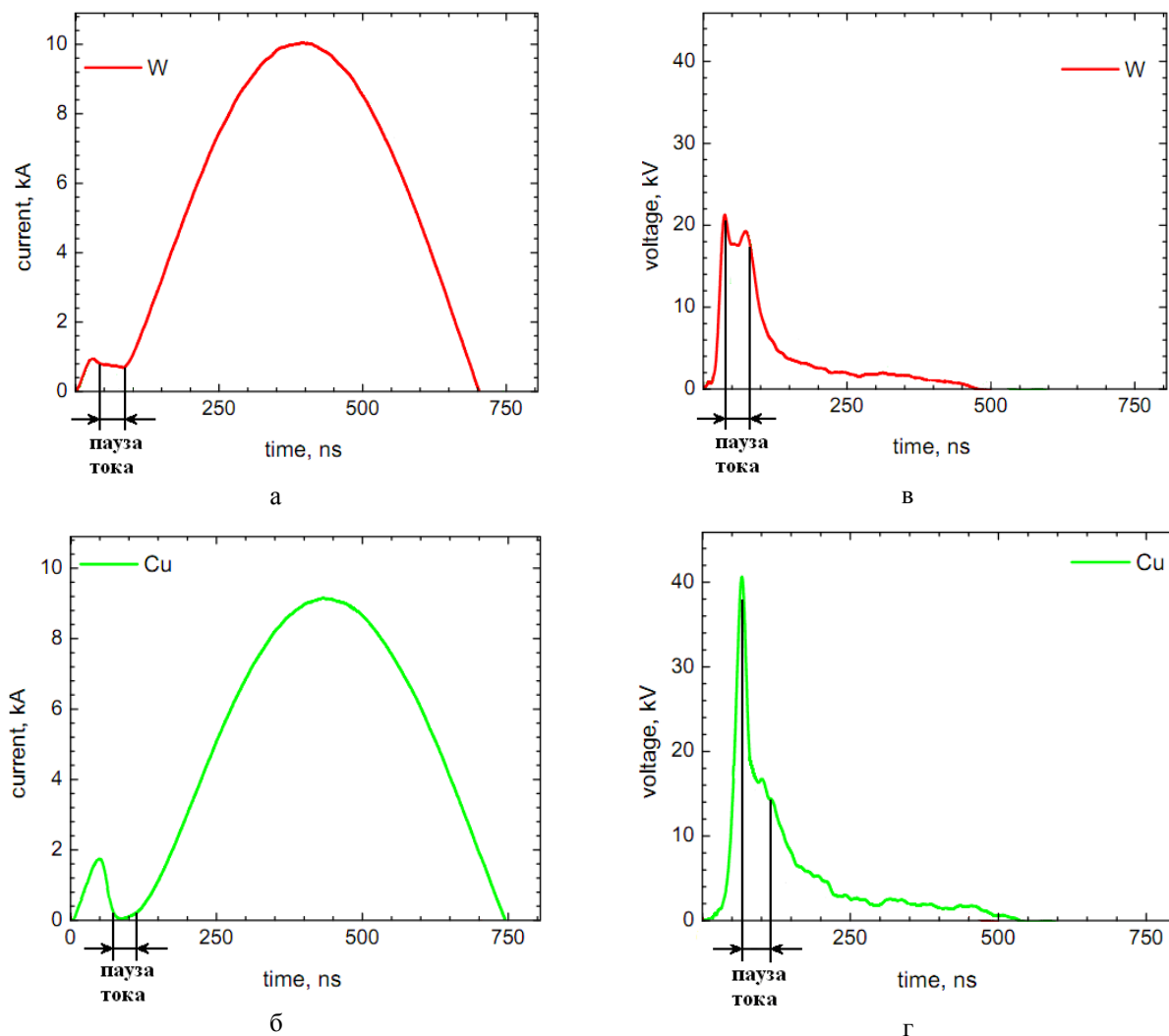
Рис. 1. Осциллограммы тока (а, б) и напряжения (в, г) при электрическом взрыве вольфрамового (а, в) и медного (б, г) проводников диаметром 0,025 \cdot 10^{-3} м и длиной 12 \cdot 10^{-3} м с учетом возникновения паузы тока и вторичного пробоя
