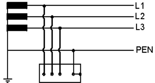
Рис. 3. Система організації мережі електроживлення за схемою TN-C
