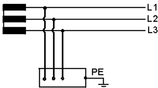
Рис. 2. Система організації мережі електроживлення за схемою IT
