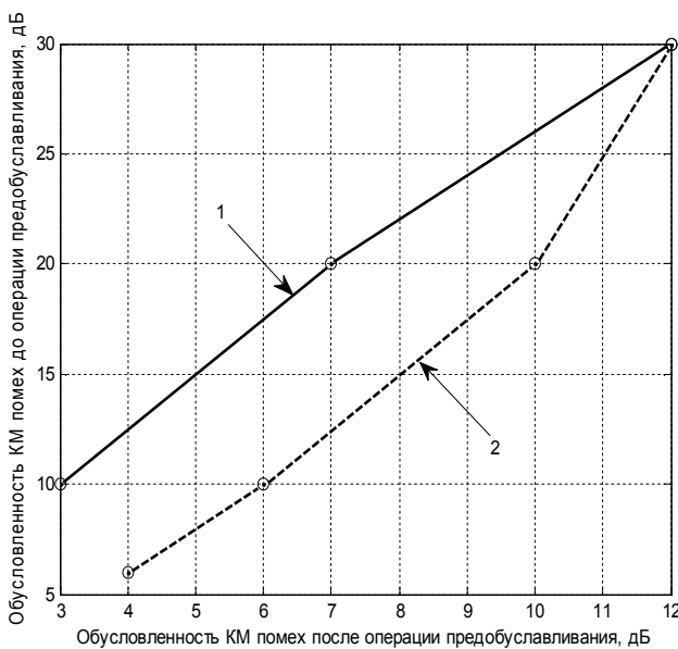
Рис. 2. Значения обусловленности КМ помех после операции предобумовлювания: 1 – N=2 ; 2 – N=4
