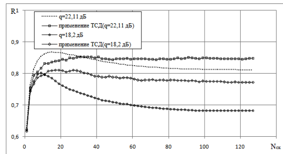
Рис. 4. Зависимости коэффициента корреляции R между оригинальным (без шума) \mathbf{X} и восстановленным изображением \mathbf{X}_{сурр}(N_{СК}) = \mathbf{X}_{И.ТСД}(N_{СК})
