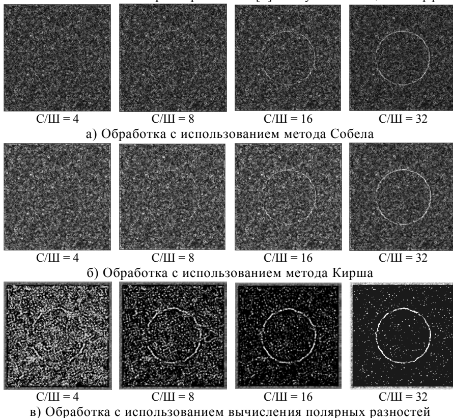
Рис. 3. Результаты выделения контуров тестовых изображений
