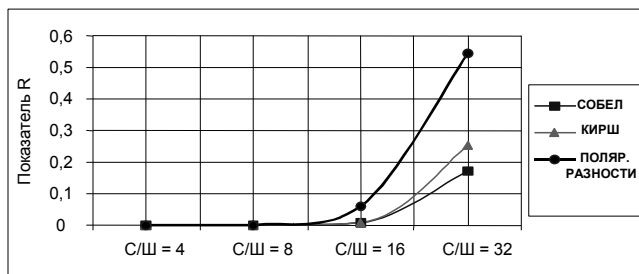
Рис. 4. Зависимость R(h) для известных методов выделения контуров
