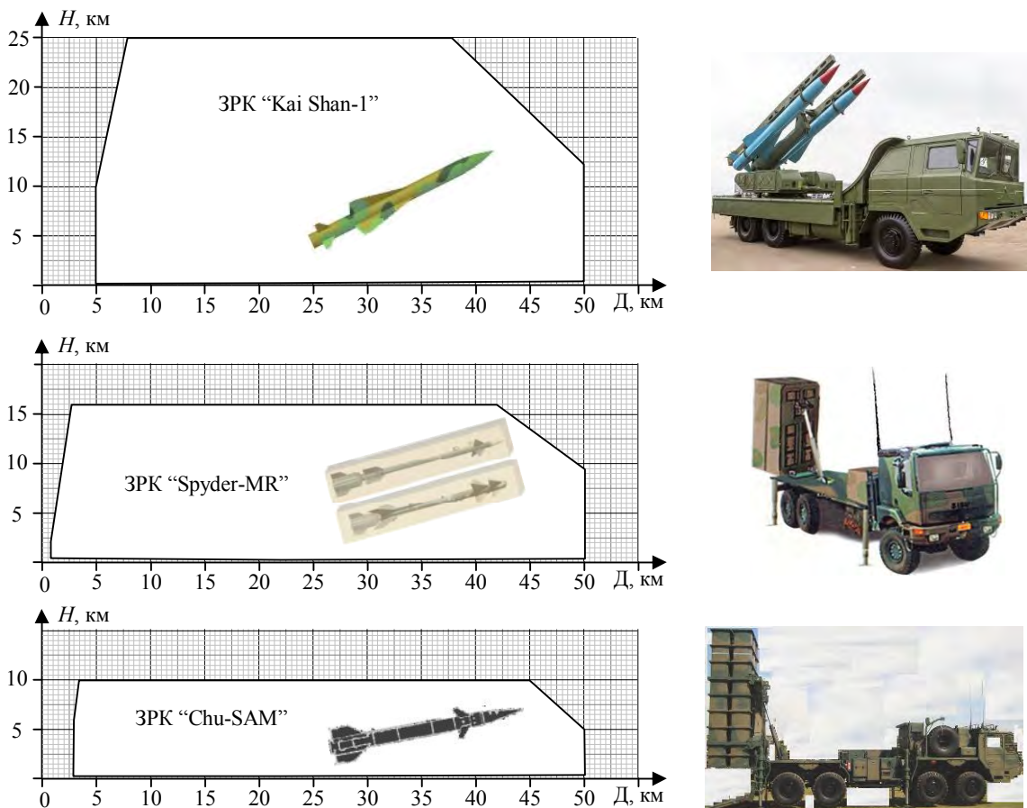
Рис. 8. Вертикальний переріз зон поразення ЗПК СД аеродинамічних цілей ( V_{ц} = 300 м/с)
