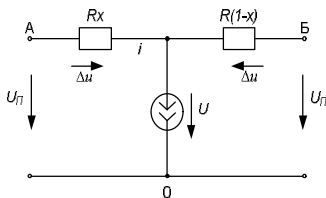
Рис. 2. Еквівалентна схема міжпідстанційної ділянки: u_n – напруга на підстанціях; R – активний опір; P – потужність ЕРС, що рухається; x – відносна відстань
