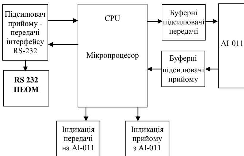
Рис. 1. Схема пристрою для спряження АПД АІ-011 з ПЕОМ
