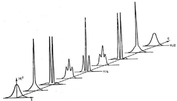
Рис. 1. Самоствиск N -солітонового імпульсу при нерезонансному самовпливові у волоконному світловоді ( N = 4 )
