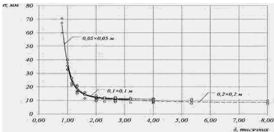
Рис. 5. Залежність СКВ координат наведення прицілу PSO-1 від уявних куткових розмірів цілі
