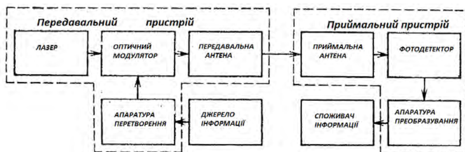
Рис. 1. Структурна схема однобічної системи ЛОЗ
